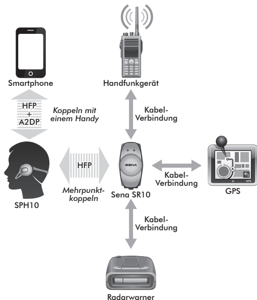
Parallele Verbindung des SR10 und des Handys per Bluetooth-Mehrpunkt-kopplung
